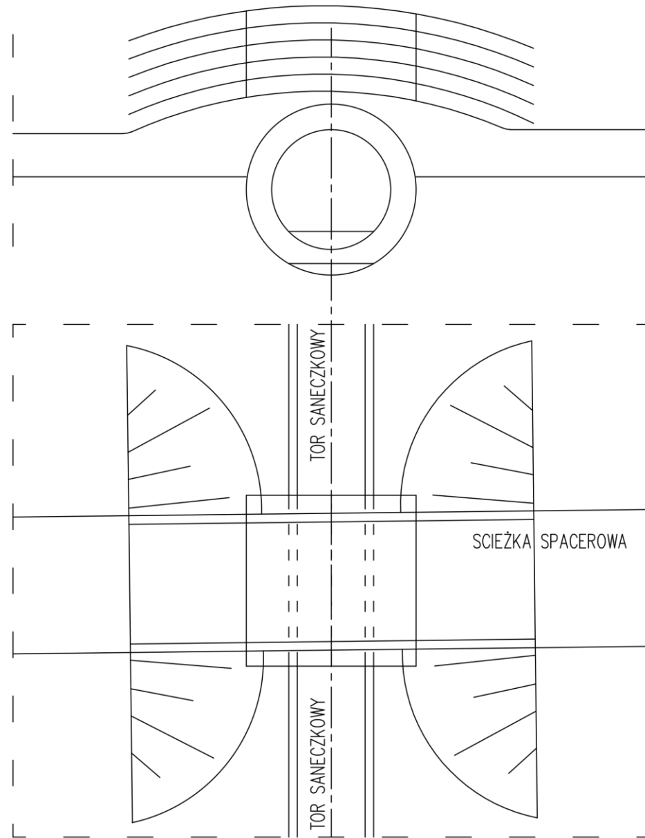
PŮDORYS A ŘEZ SÁŇKAŘSKÉ DRÁHY / RZUT I PRZEKRÓJ TORU SANECZKOWEGO
