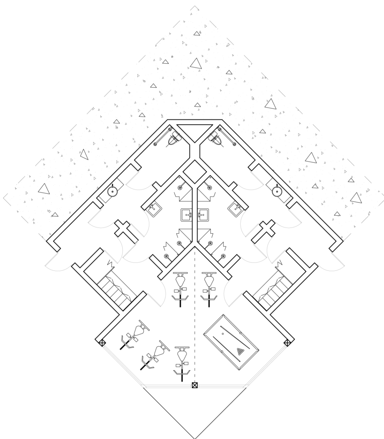
PŪDORYS PAVILONU / PLAN PAWILONU
